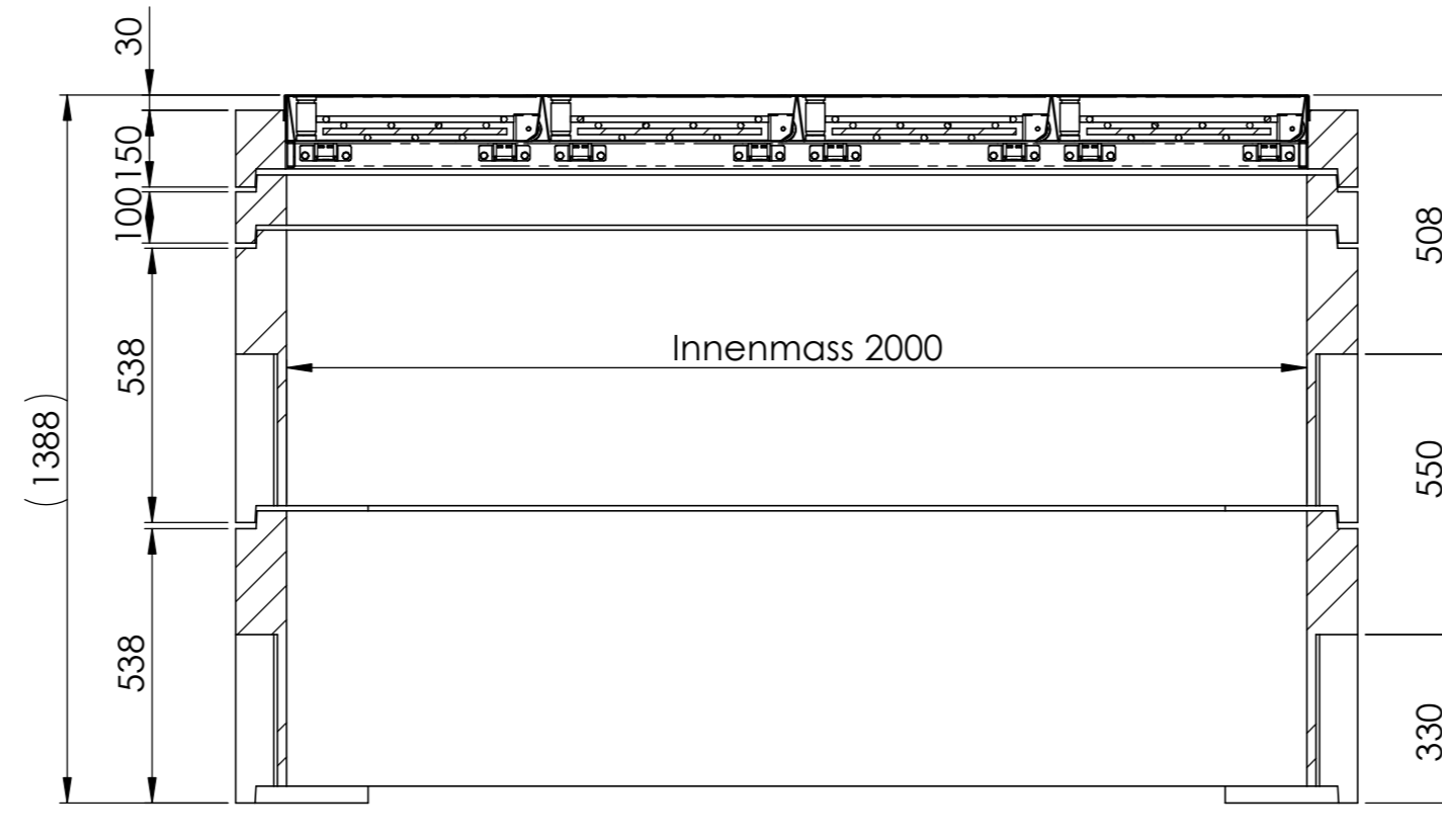
SCHNITT A-A MABSTAB 1:15
